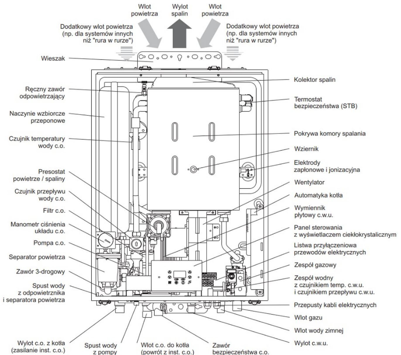
SCHEMAT ROZRZUCONY KOTŁA ULRICH WANDICH FUTURA PLUS
