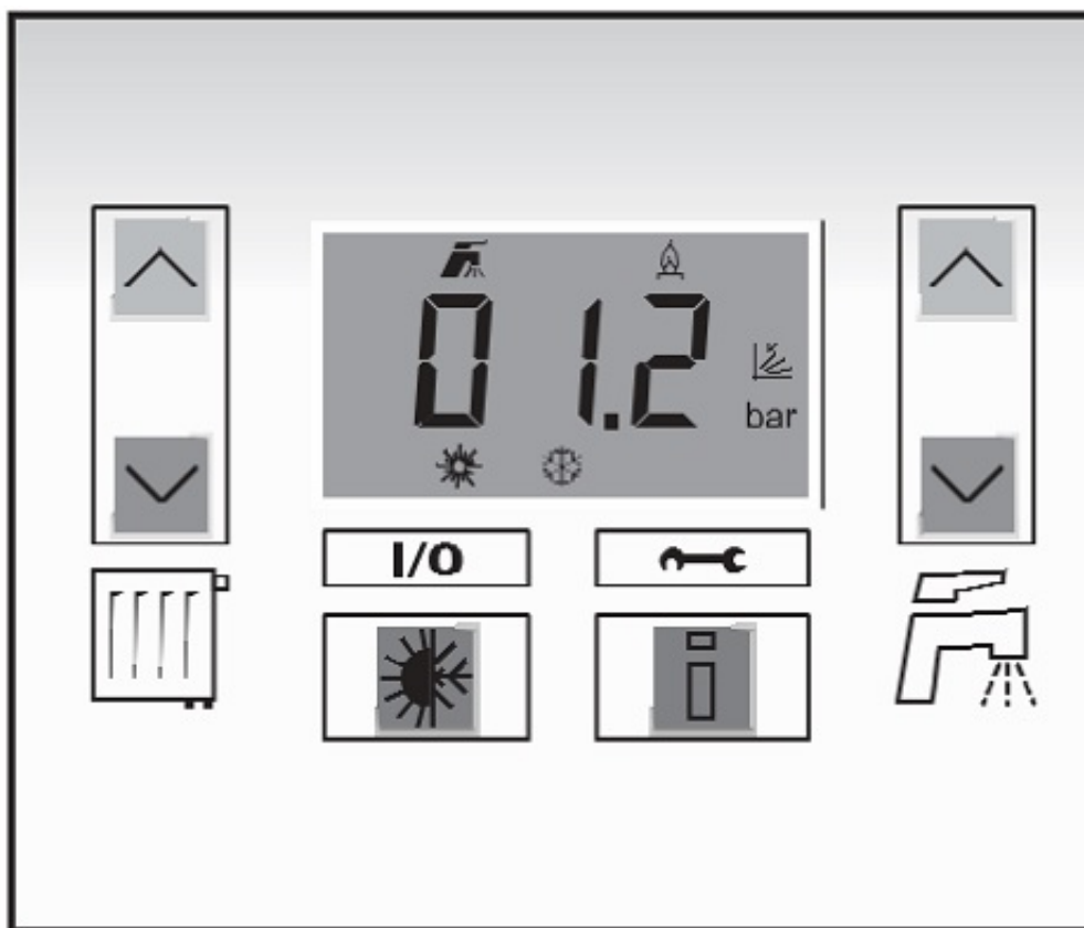
Panel wyświetlacza LCD w obudowie kotła
