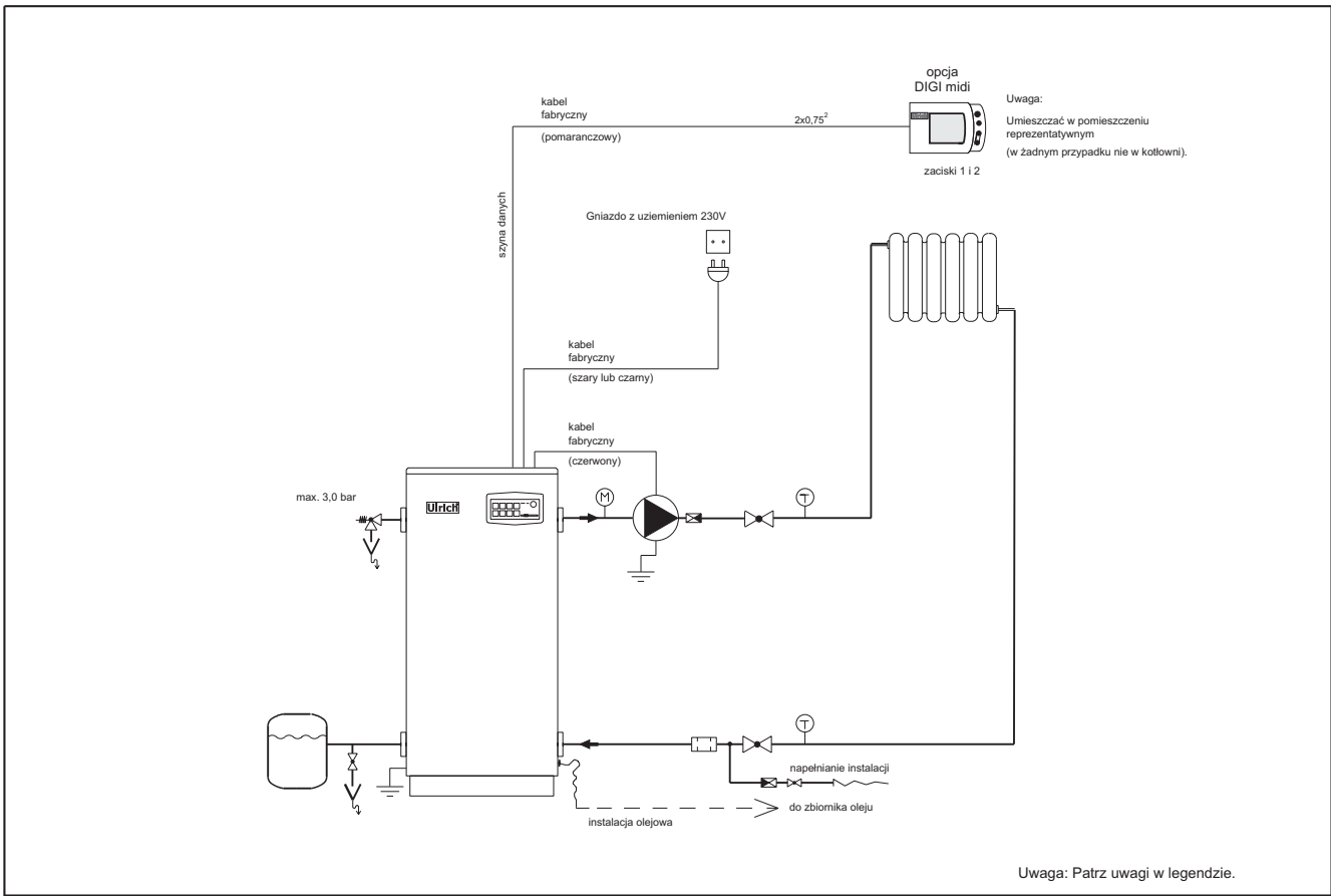
©Ulrich Ver. 09.2010 Rys. 04 Kocioł w zestawie Wertich Oil WO... - podstawowy schemat, instalacja ciśnieniowa. Ulrich
