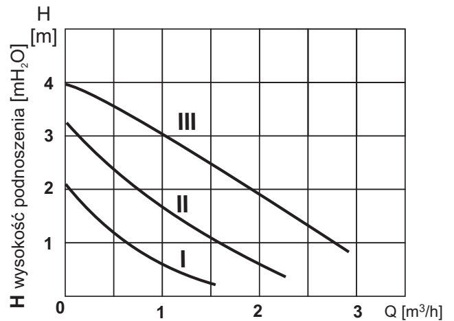
Q przepływ [m³/h] Rys. Charakterystyka pompy
