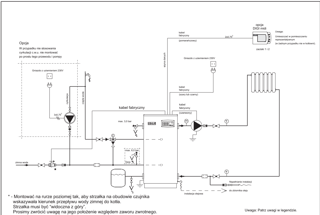
©Ulrich Ver. 09.2010 Rys. 05 Kocioł w zestawie Wertich Oil WO...+W - podstawowy schemat, instalacja ciśnieniowa. Ulrich
