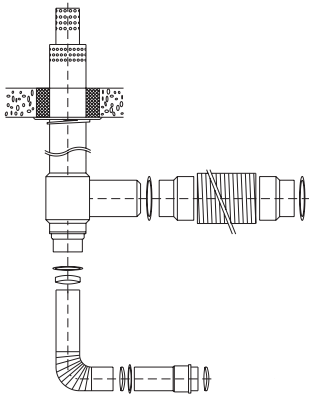
System spalinoowo-powietrzny typu "turbo" -typowy
