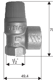
Rys. Wymiary zaworu
